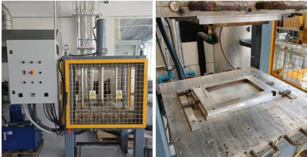
Prensa utilizada para la realización de los materiales compuestos polímero-partícula sacado de la prensa
